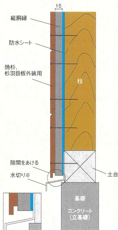
焼杉、杉羽目板外装用（横張り）施工図
