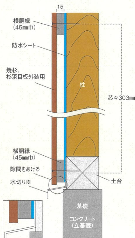
焼杉、杉羽目板外装用（縦張り）施工図
